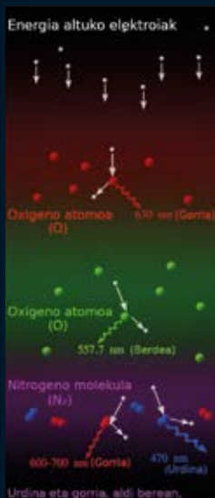
3. irudia. Atmosferara heltzen diren partikula kargadunen eta molekula ezberdinekin talkan sortzen dituzten trantsizio eta koloreen irudikapena. Kredituak: https://www.lwpetersen.com/science-and-nature/what-causes-the-aurora/
