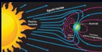
1. irudia. Eguzki-haizearen (ur-dinez) eta Lurraren eremu magnetikoaren (gorriz) irudikapena. Kredituak: University of Waikato ( www.sciencelearn.org.nz )
