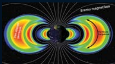
2. irudia. Lurraren eremu magnetikoa (zuriz) eta Van Allenen gerrikoak (koloreek partikula kargadunen dentsitatea adieraztzen dute, dentsitate maximoa gorria delarik). Irudia: Kredituak: Houston Space Center ( https://spacecenter.org/what-are-the-van-allen-radiation-belts/ )
